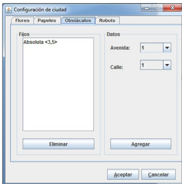
Figura 4.4. Configurar obstáculos
