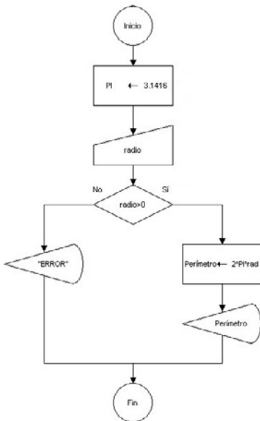
Proceso Problema3
